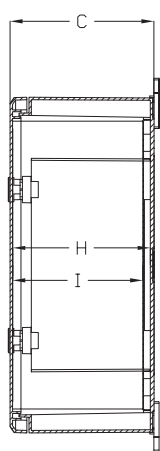
CORTE A-A
