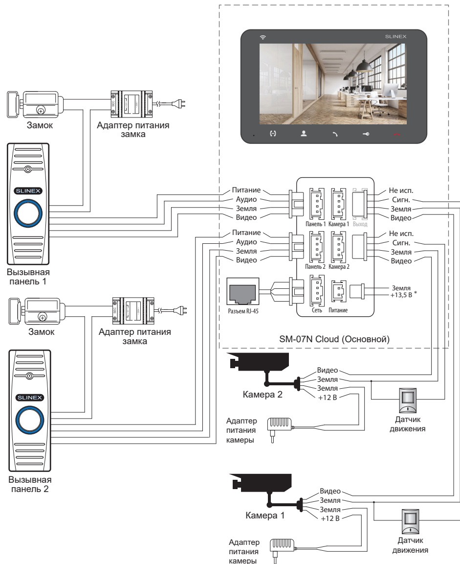
Схема 1. Подключение вызывных панелей и камер к домофону SM-07N Cloud.
